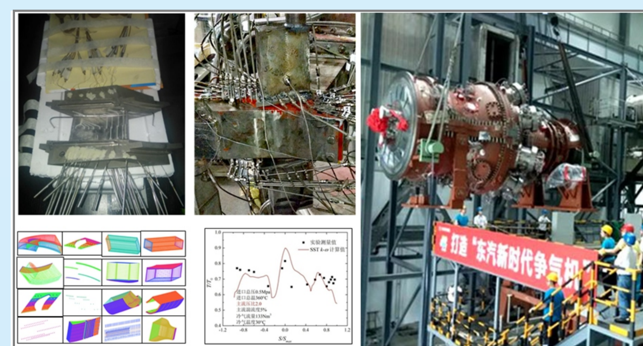
重型燃气轮机第一级导叶的冷效可靠性设计
